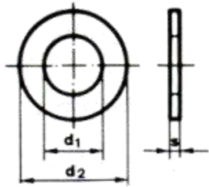
DIN 125 A Flat washer without chamfer
