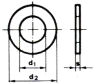
DIN 126 Flat washer without chamfer
